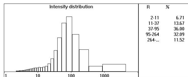
Рис. 1. Усредненная ЛКС-гистограмма плазмы крови здоровых доноров.
